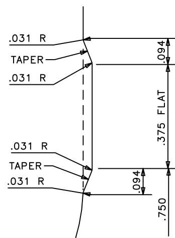
SECTION B-B SCALE: 4 TO 1
