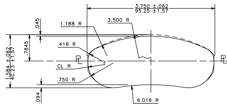
TYP SECTION THRU BODY
